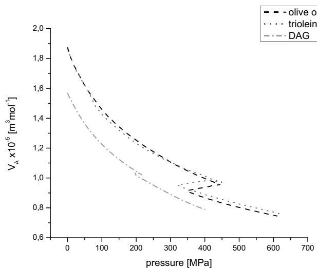
Fig. 9 Parameter V_A vs pressure at 20 °C
